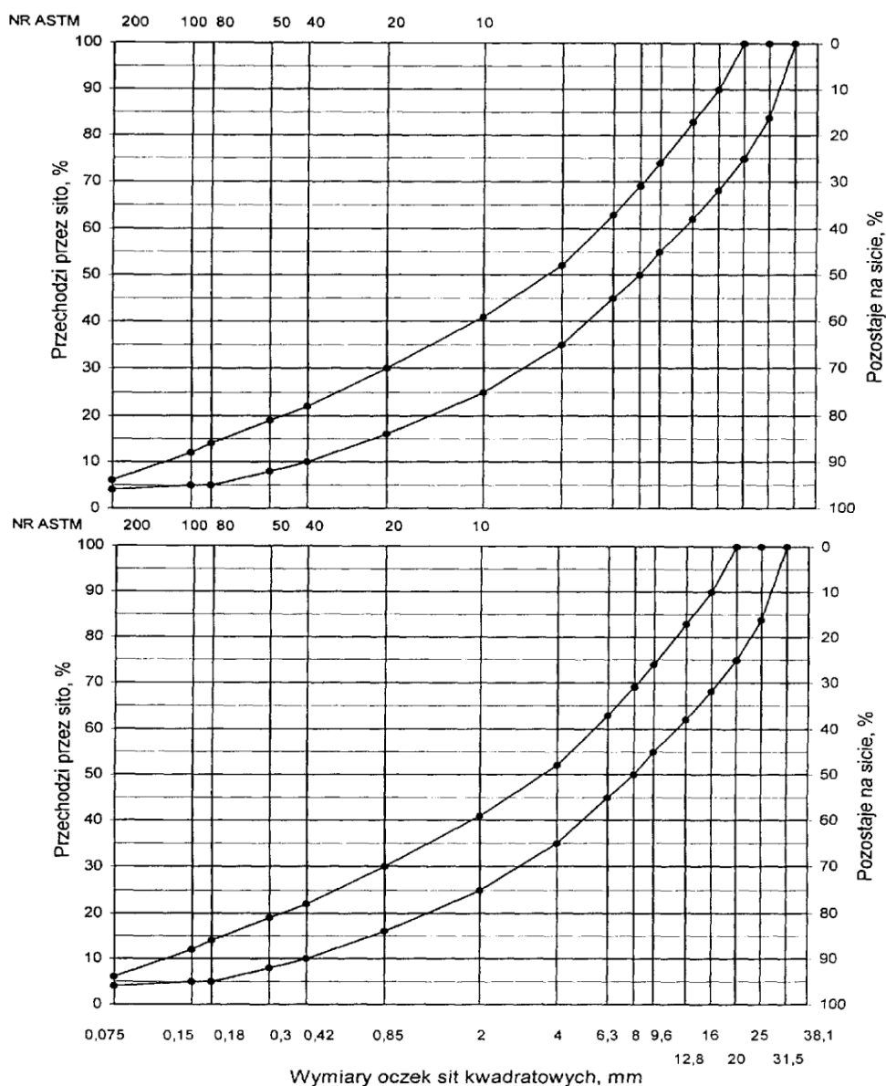
Rys. 11. Krzywe graniczne uziarnienia mieszanki mineralnej BA od 0 do 25 mm do warstwy wiążącej, wyrównawczej i wzmacniającej nawierzchni drogi o obciążeniu ruchem od KR3 do KR6 Rys. 12. Krzywe graniczne uziarnienia mieszanki mineralnej BA od 0 do 20 mm do warstwy wiążącej, wyrównawczej i wzmacniającej nawierzchni drogi o obciążeniu ruchem od KR3 do KR6
