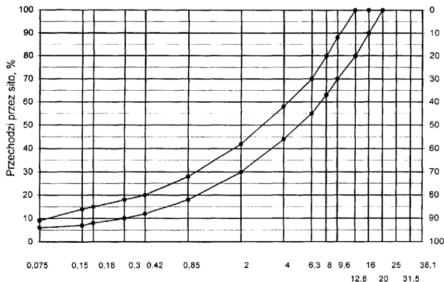
Rys. 6. Krzywe graniczne uziarnienia mieszanki mineralnej BA od 0 do 16 mm do warstwy ścieralnej nawierzchni drogi o obciążeniu
