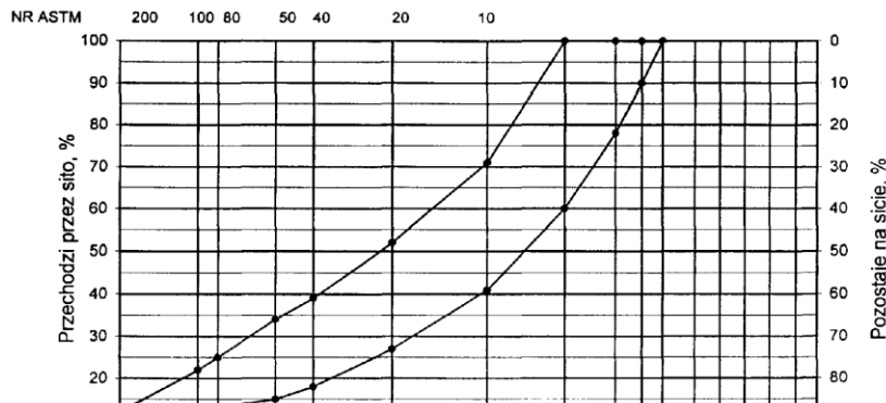
Rys. 3. Krzywe graniczne uziarnienia mieszanki mineralnej BA od 0 do 8mm, od 0 do 6,3 mm do warstwy ścieralnej nawierzchni drogi o obciążeniu ruchem nawierzchni drogi o obciążeniu ruchem KR1 lub KR2
