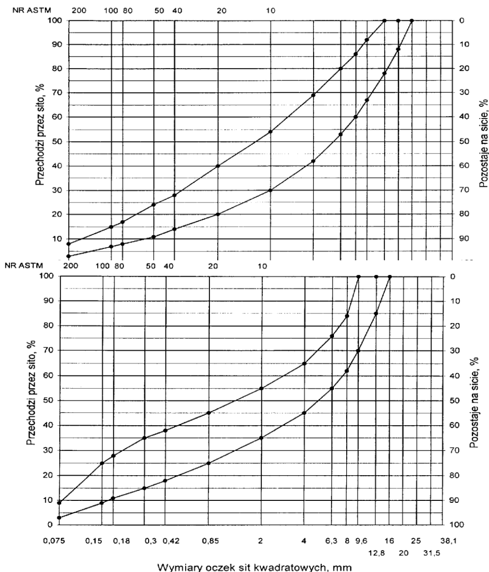
Rys. 10. Krzywe graniczne uziarnienia mieszanki mineralnej BA od 0 do 12,8 mm do warstwy wiążącej, wyrównawczej
