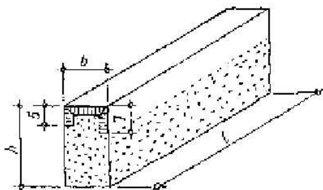
Rys. 6. Krawężnik drogowy rodzaju B
